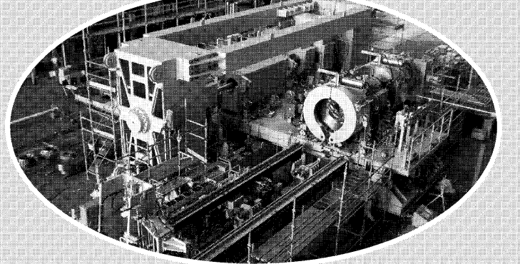
「高水圧」「高精度」による「複合水圧試験機」[Collapse and Bursting Tester]
