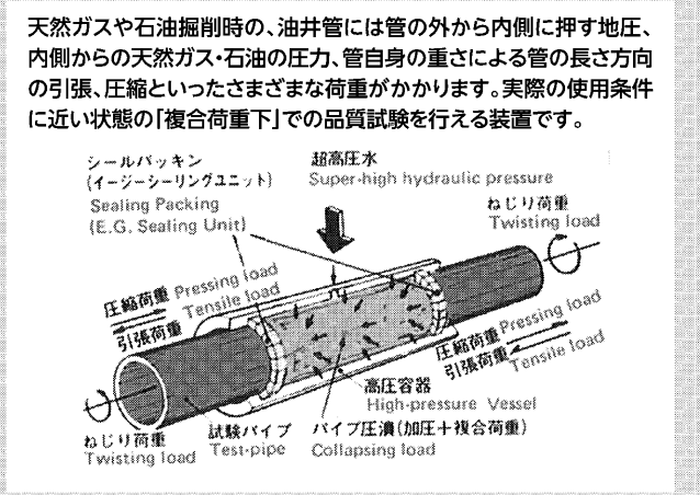
「高水圧」「高精度」による「複合水圧試験機」[Collapse and Bursting Tester]
